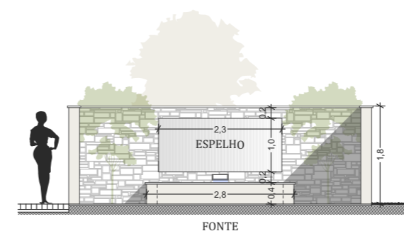
Corte - Patio
