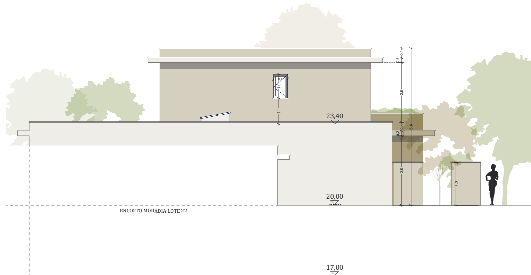
Alçado Norte
