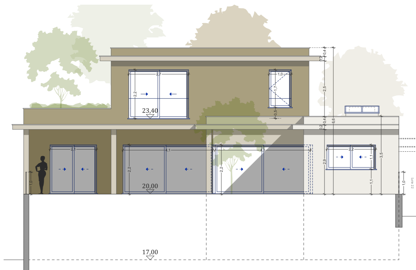
Alçado Este
